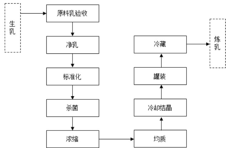
图 A.3 炼乳典型工艺流程图
