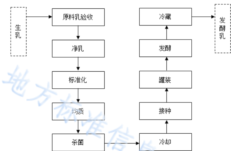
图 A.4 全脂发酵乳典型工艺流程图
